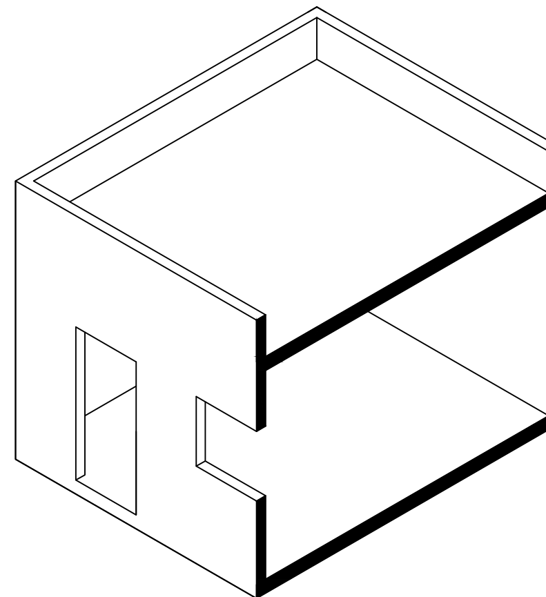
ISOMETRÍA CORTE C-C'
